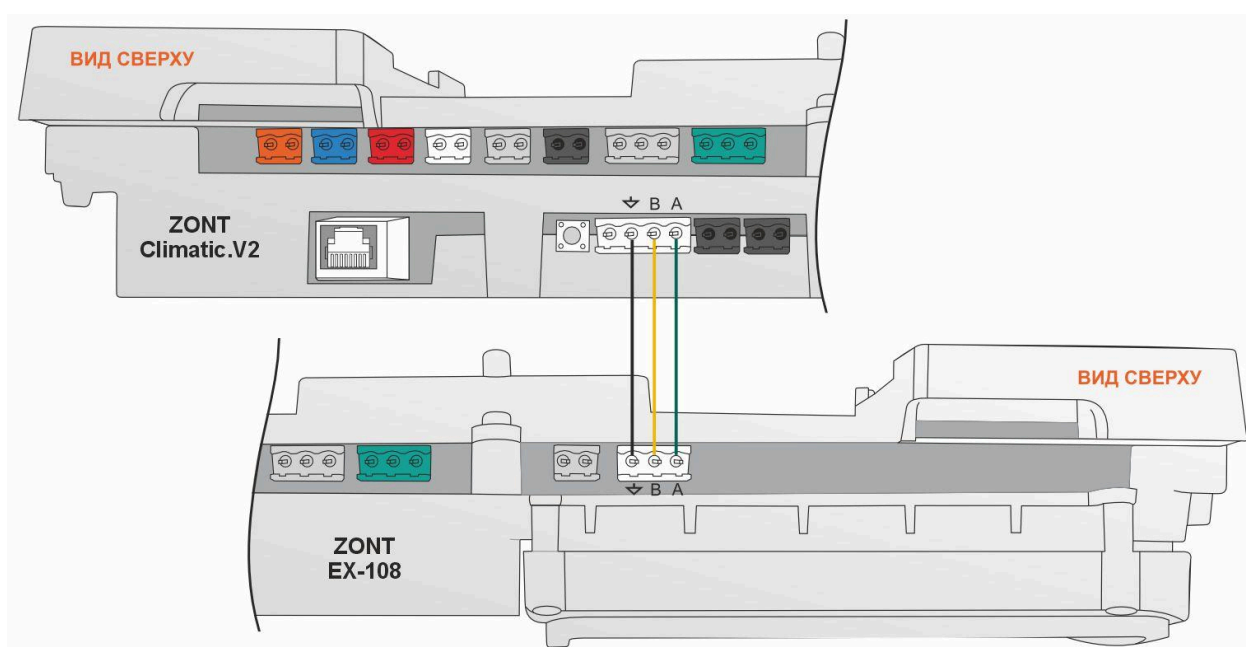
Схема подключения блока расширения EX-108
